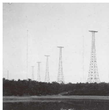
小野受信所のアンテナ (昭和51年ごろ)
