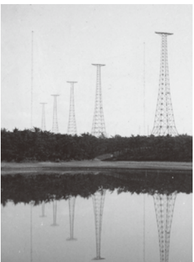
小野受信所のアンテナ(昭和51年ごろ)
