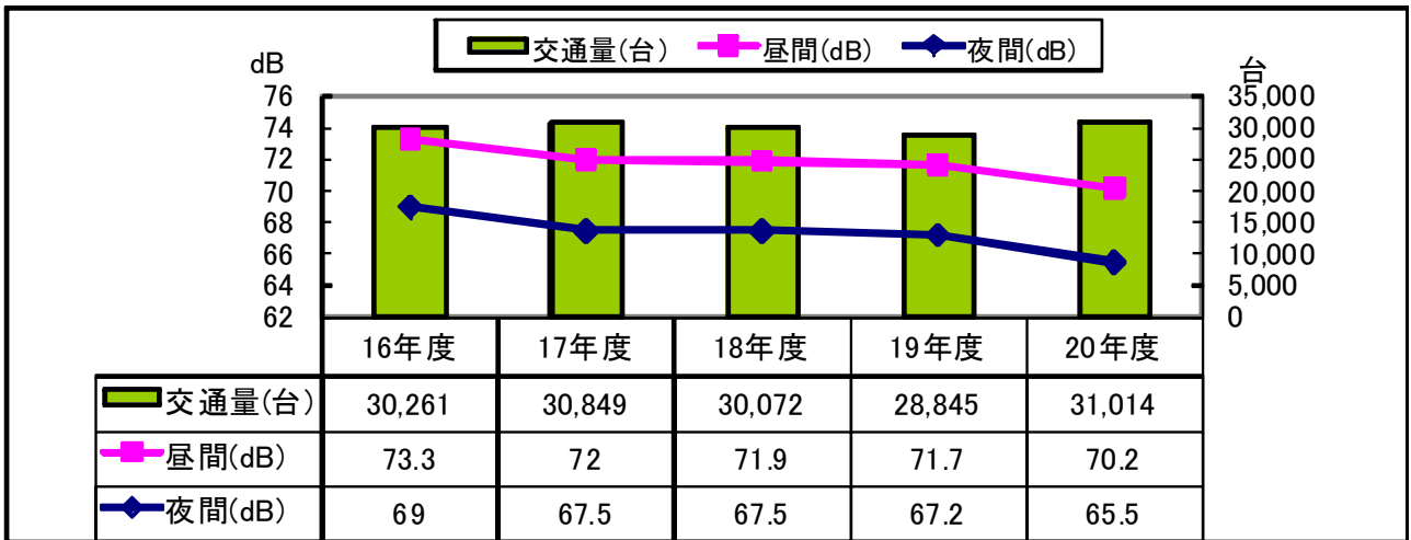
国道175号線 交通騒音と交通量の経年比較
