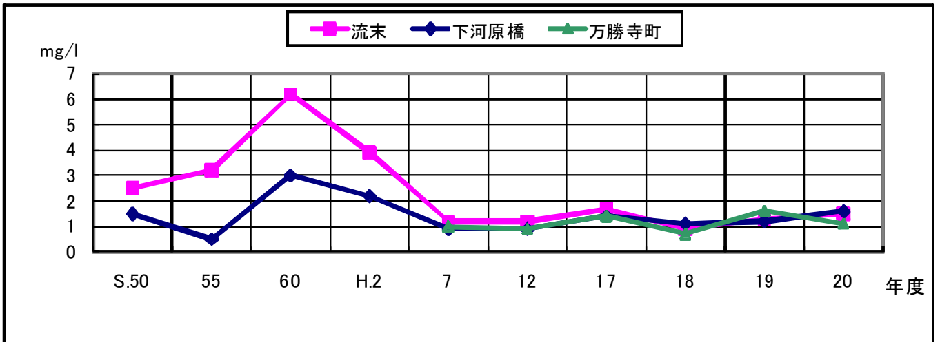
BOD 経年変化（万勝寺川）
