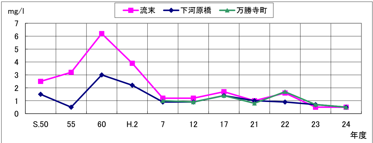
BOD 経年変化（万勝寺川）
