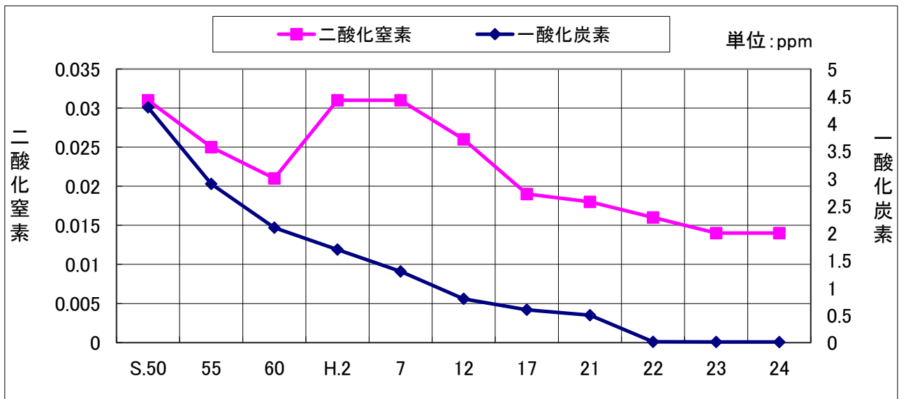
道路環境測定結果経年変化（県道小野加古川線・上本町自動測定所）
