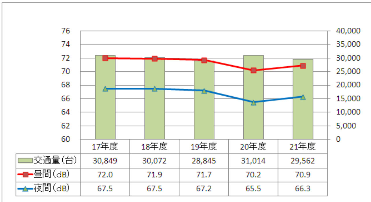
国道175号線 交通騒音と交通量の経年比較
